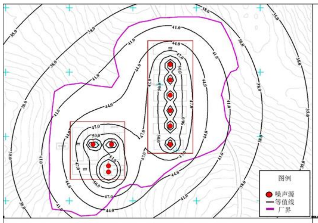
图 12-1 黄陂稀土矿富集站一厂界噪声预测结果
