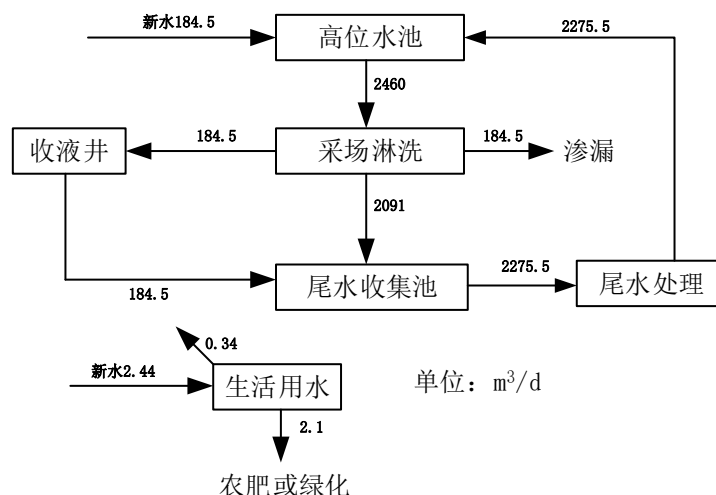
图 4-12 黄陂稀土矿只有清水淋洗期水平衡图
