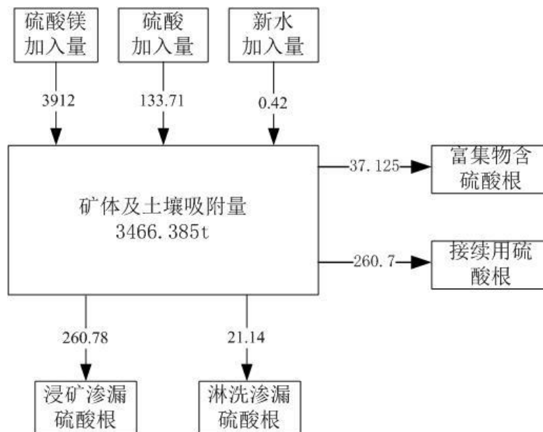
图 4-13 硫酸盐平衡图
