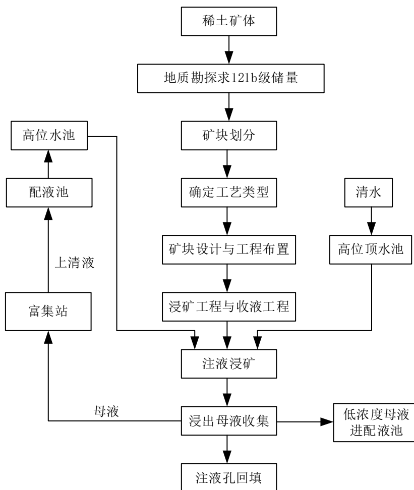
图 4-5 原地浸矿工艺流程图
