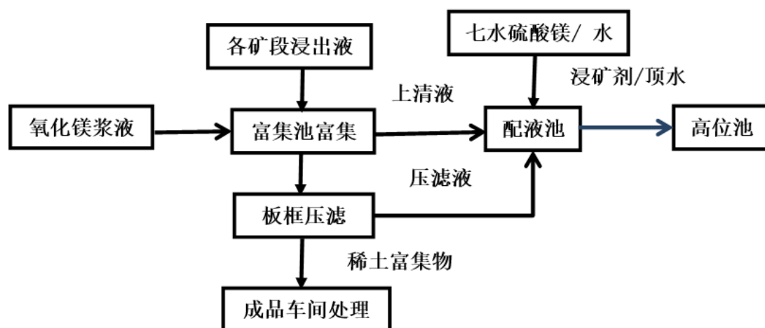
图 4-9 黄陂稀土矿母液处理工艺流程图
