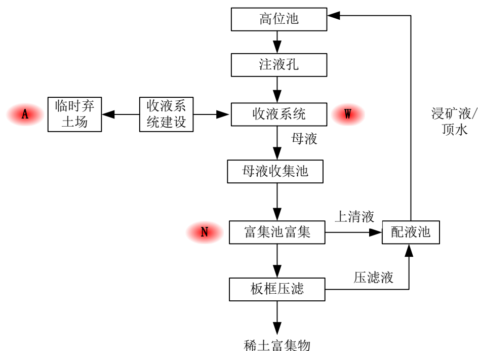
图 4-15 原地浸矿主要污染源发生点位图
