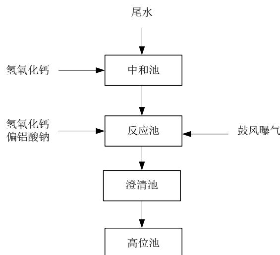
图 4-16 钙矾石法工艺流程图
