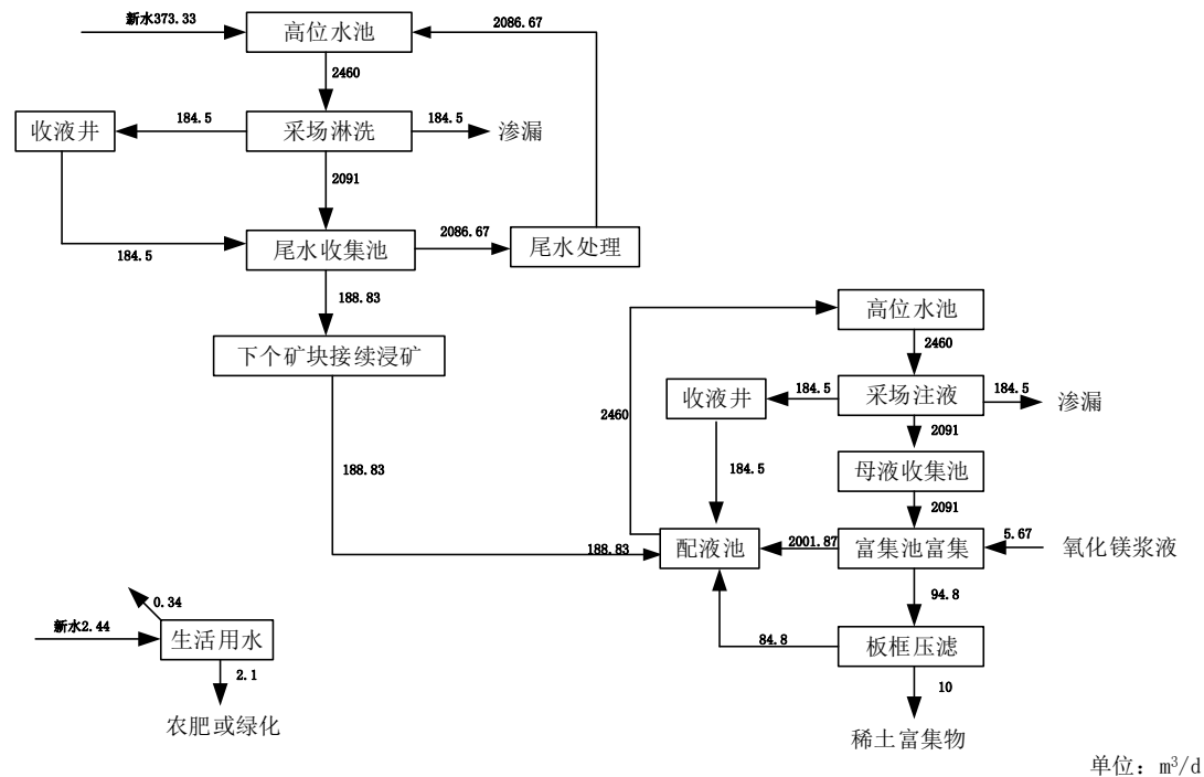
图 4-11 黄陂稀土矿生产期及清水淋洗期水平衡图
