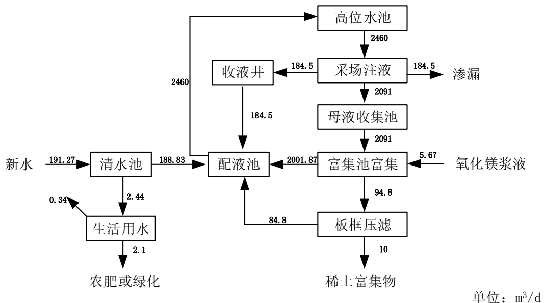
图 4-10 黄陂稀土矿生产期水平衡图
